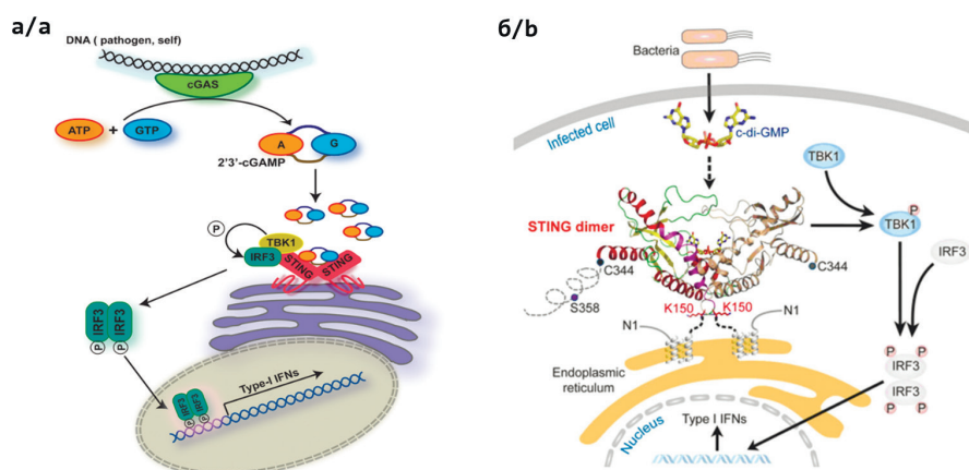
Рис. 1. Сигнальные пути, реализуемые с участием эффектора млекопитающих cGAS (а) и его бактериального аналога c-di-GMP (б) [5].
