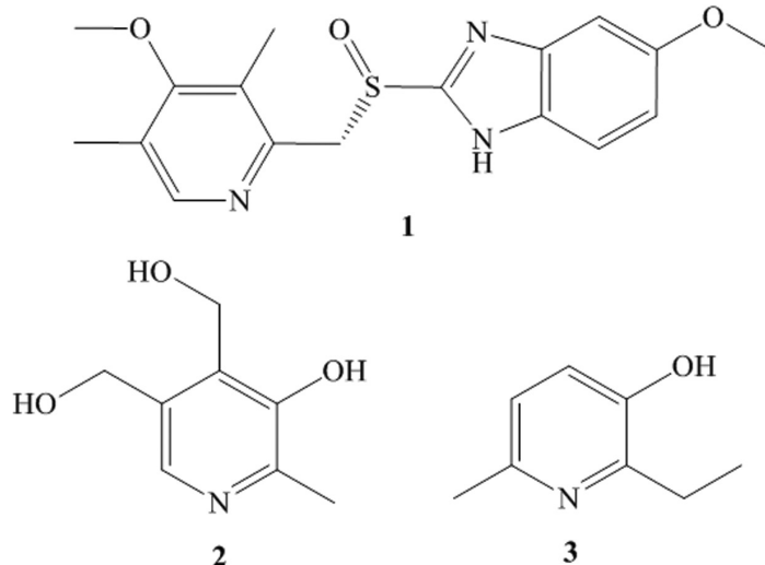
Рис. 1. Структурные формулы эзомеразола 1 , пиридоксина 2 и эмоксипина 3
