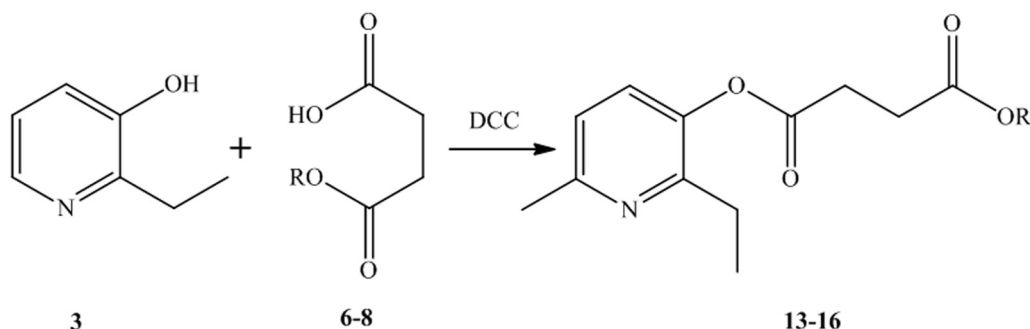
Рис. 3. Ацилирование эмоксипина 3 моноэфирами янтарной кислоты
